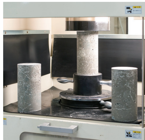
圧縮試験機
